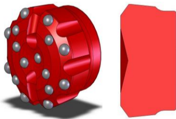
Cara Cóncava
